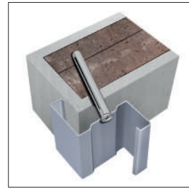
Installazione telaio avvitato a muro
