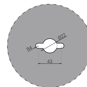
FORO MANIGLIA
