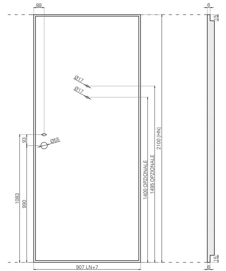
SICURA PRO LATO ESTERNO
