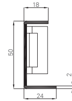
ESEMPIO PORTA SICURA PRO 900X2100 CON FALSO TELAIO SUPER RIDOTTO
