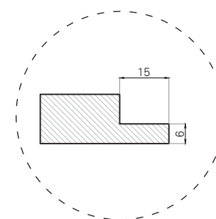
BATTUTA PERIMETRALE
