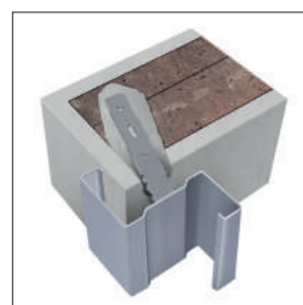
Installazione telaio zancato a muro
