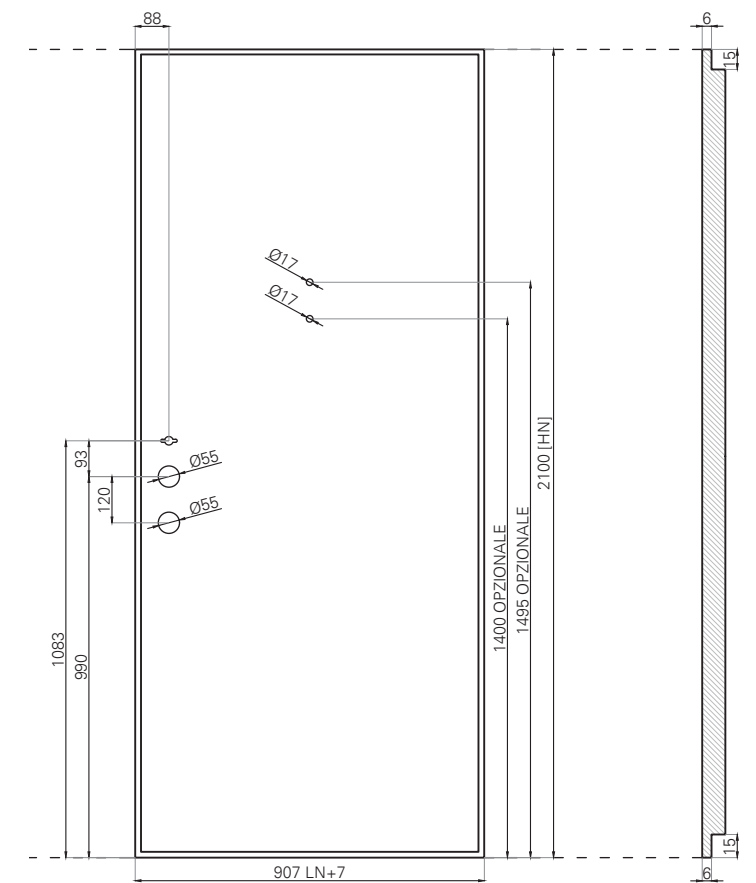
SICURA MI PRO LATO ESTERNO
