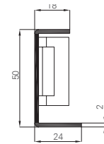
ESEMPIO PORTA SICURA MI PRO 900X2100 CON FALSO TELAIO SUPER RIDOTTO
