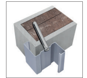
Installazione telaio avvitato a muro
