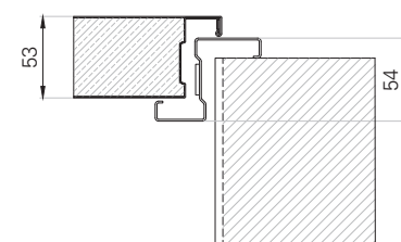
Dettaglio sezione orizzontale
