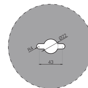
FORO MANIGLIA
