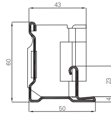
ESEMPIO PORTA SICURA PRO 900X2100 CON FALSO TELAIO STANDARD
