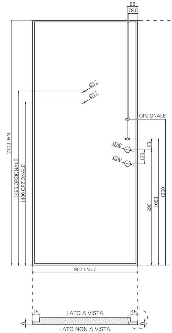
SICURA MI PRO LATO INTERNO
