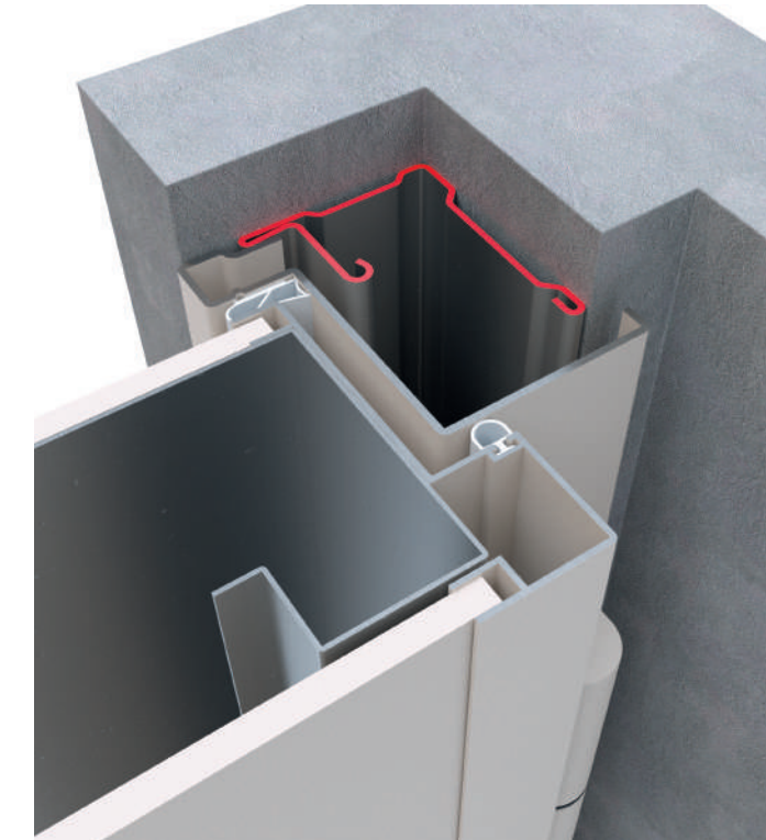
FALSO TELAIO SUPER RIDOTTO
