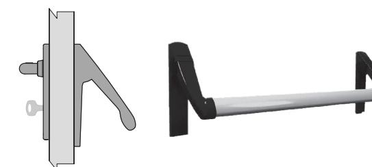
Kit maniglione antipanico Tecno a leva sporgenza 110 mm (base nera / barra alluminio) + 1/2 maniglia standard lato a tirare + 1/2 cilindro esterno Serratura antipanico compresa
