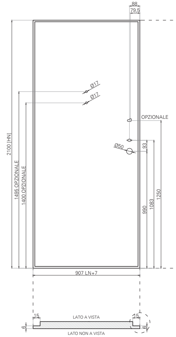
SICURA PRO LATO INTERNO
