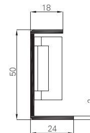
SEZIONE A-A
