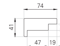
DETTAGLIO TECNICO
