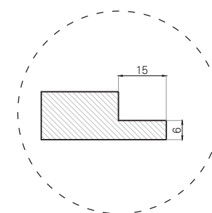
BATTUTA PERIMETRALE
